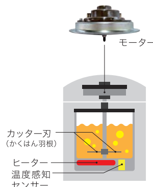
⑨クックマスター 旬彩Pro YE-CM17B
