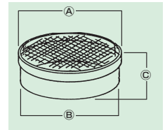
裏漉・絹漉の寸法表・図
