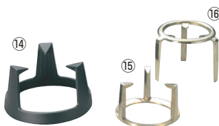
⑭SE 鉄イモノ 三つ足 五徳 外寸 商品コード 価格 E-73 大 φ247×H145 6058900 ¥5,500 E-74 中 φ210×H122 6059000 ¥5,000 E-75 小 φ185×H105 6059100 ¥4,500
